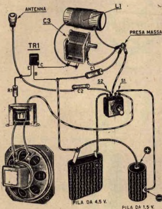
Fig. 2 - Schema pratico
