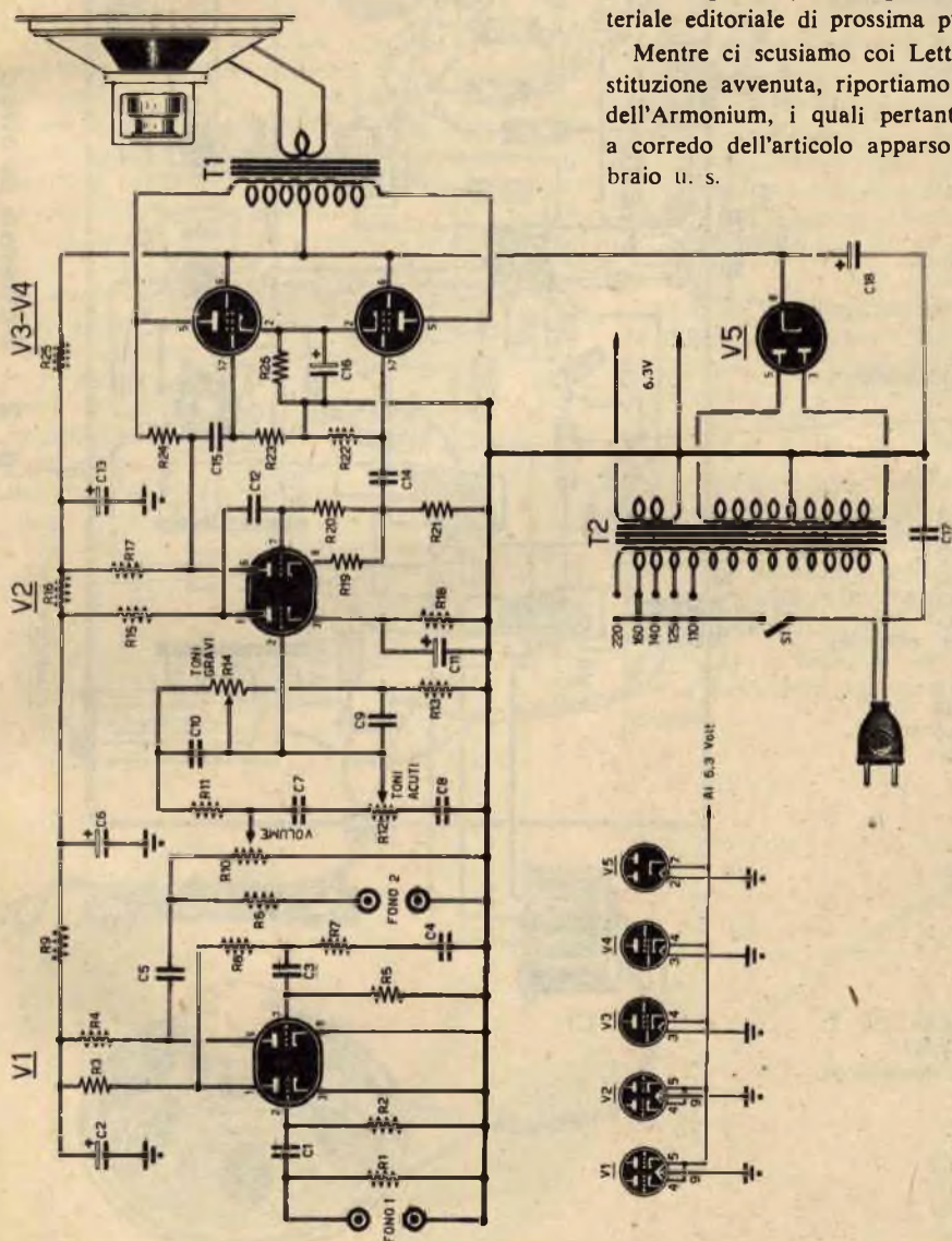
Fig. 1 - Schema elettrico
