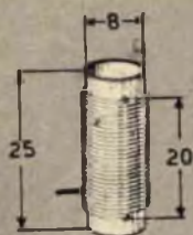
L1 24 SPIRE FILO 0,70 mm. CON PRESÀ ALLA 3ª SPIRA
