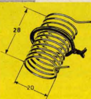
L3 1 SPIRA FILO ISOLATO AVVOLTA SU L2
