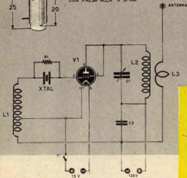
L1 24 SPIRE FILO 0,70 mm. CON PRESÀ ALLA 3ª SPIRA
