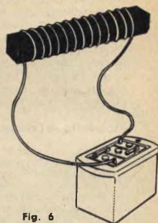
Fig. 6 - Si possono ottenere delle potenti calamite facendo circolare corrente continua in un avvolgimento a spirale di filo di rame avvolto sopra l'oggetto di acciaio da magnetizzare.
