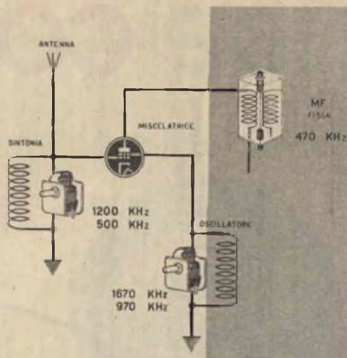
Fig. 1 - In una supereterodina si fa in modo che il condensatore variabile dell'oscillatore e quello della sintonia siano sfasati in tutta la propria corsa in modo tale da ottenere sempre all'uscita una frequenza fissa di 470 KHz.
