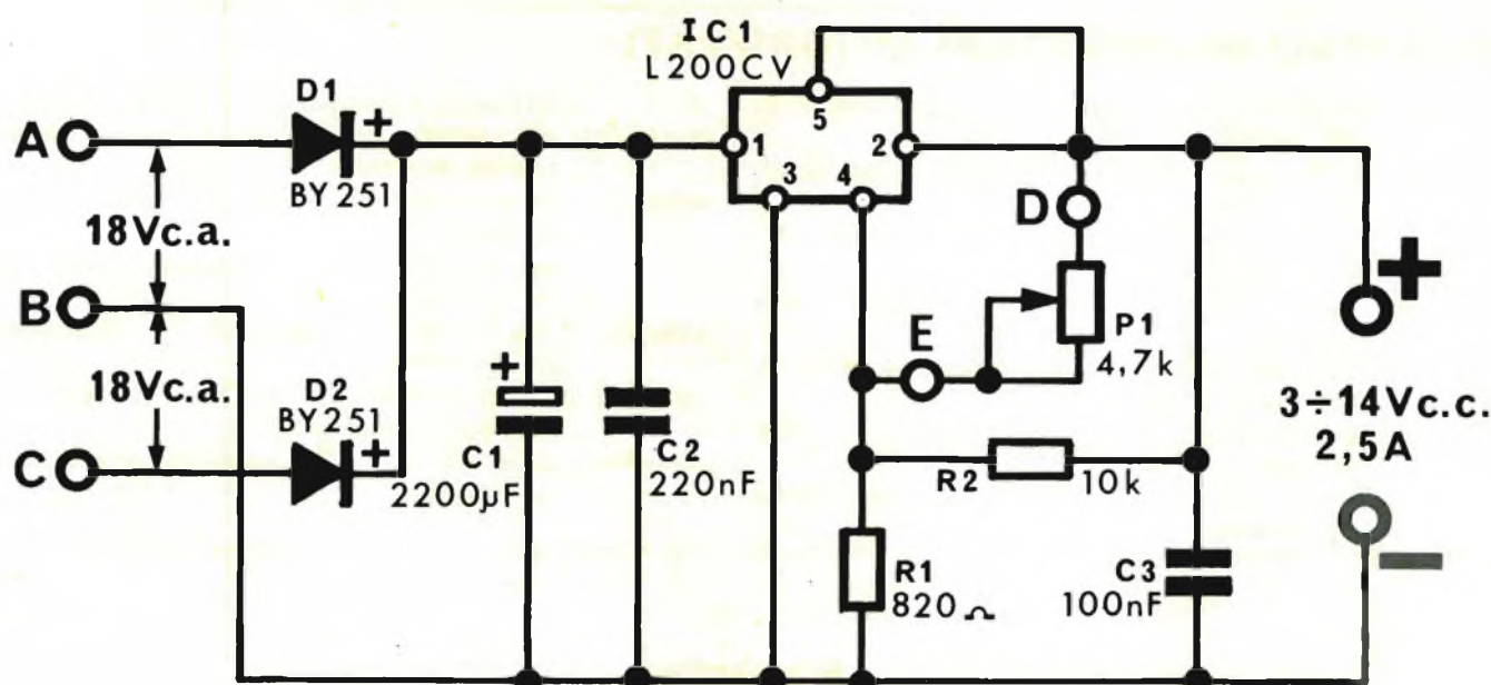
Fig. 1 - Circuito elettrico dell'alimentatore stabilizzato basato sull'integrato L200 prodotto dalla SGS.
