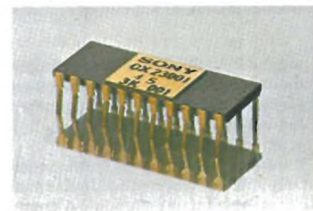
Memoria RAM in dotazione ai computer MSX della Sony. I programmi realizzati, possono essere memorizzati in uno o più di questi chip prima di togliere corrente al computer.
