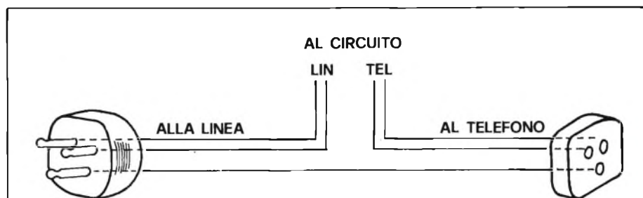
Fig. 4 - Collegamento del circuito alla linea telefonica. Molto utili si dimostrano in questo caso le spine passanti.
