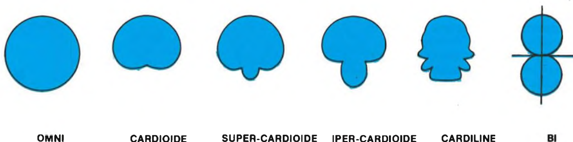
Fig. 8 - Microfono omnidirezionale.
