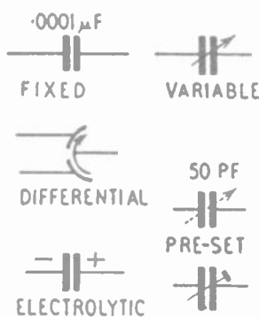
Fig. 2 Condensers
