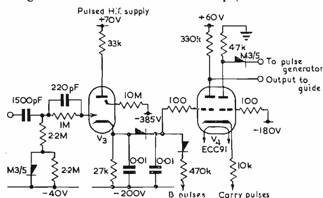
Fig. 7. Carry circuit.
